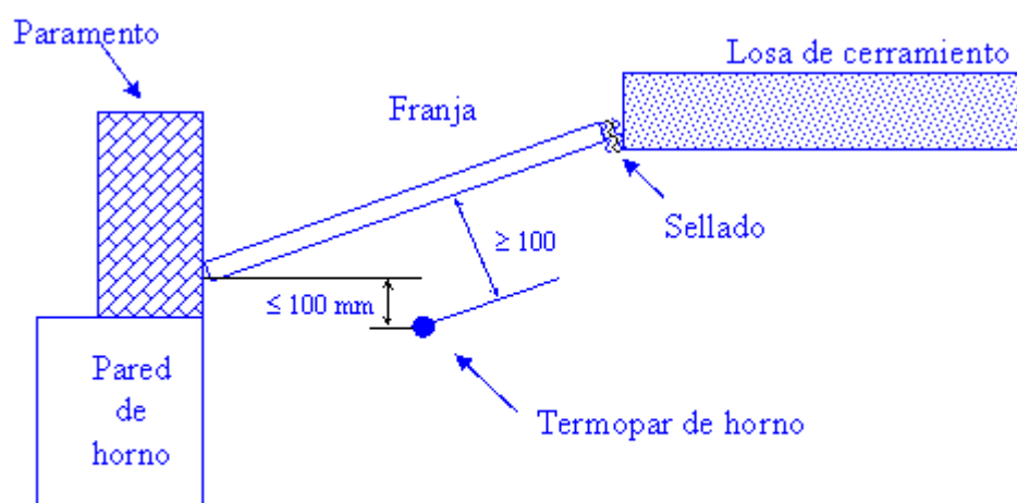
Figura 1.- Disposición Termopares de horno
